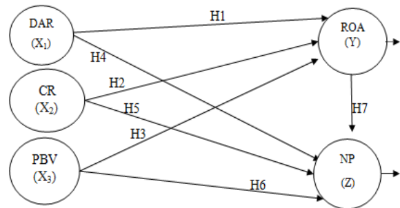
Gambar 3.1 kerangka konseptual
